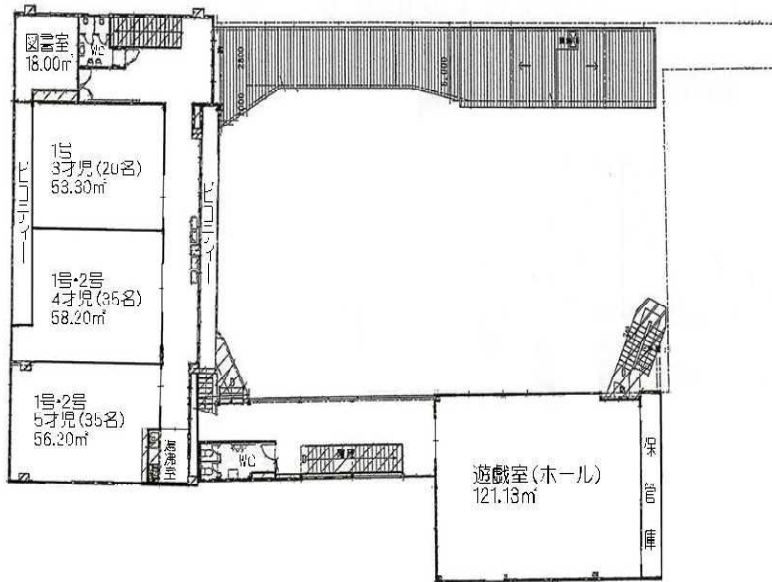
学校法人唯佛寺学園 ほうなん子ども園 平面図 (本園2階)
