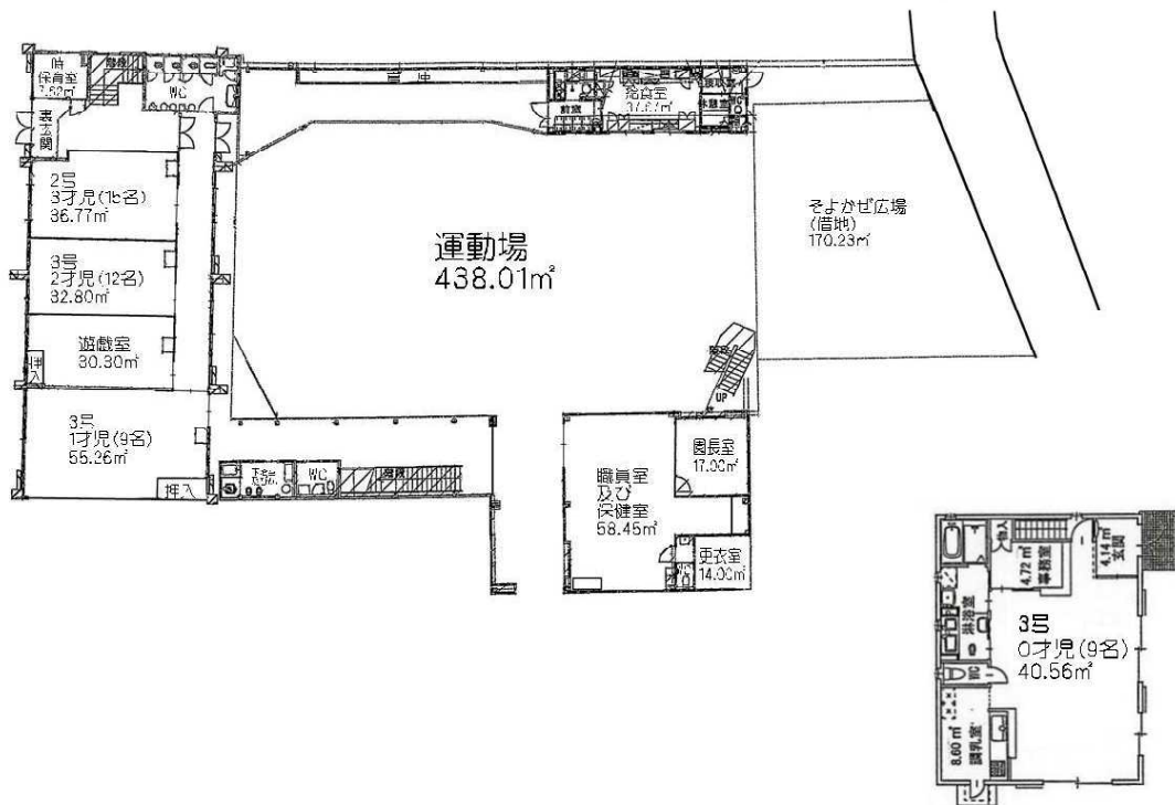
学校法人唯佛寺学園 ほうなん子ども園 平面図 (本園1階)
