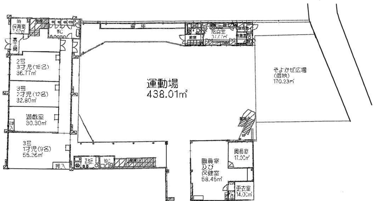
学校法人唯佛寺学園 ほうなん子ども園 平面図 (本園1階)
